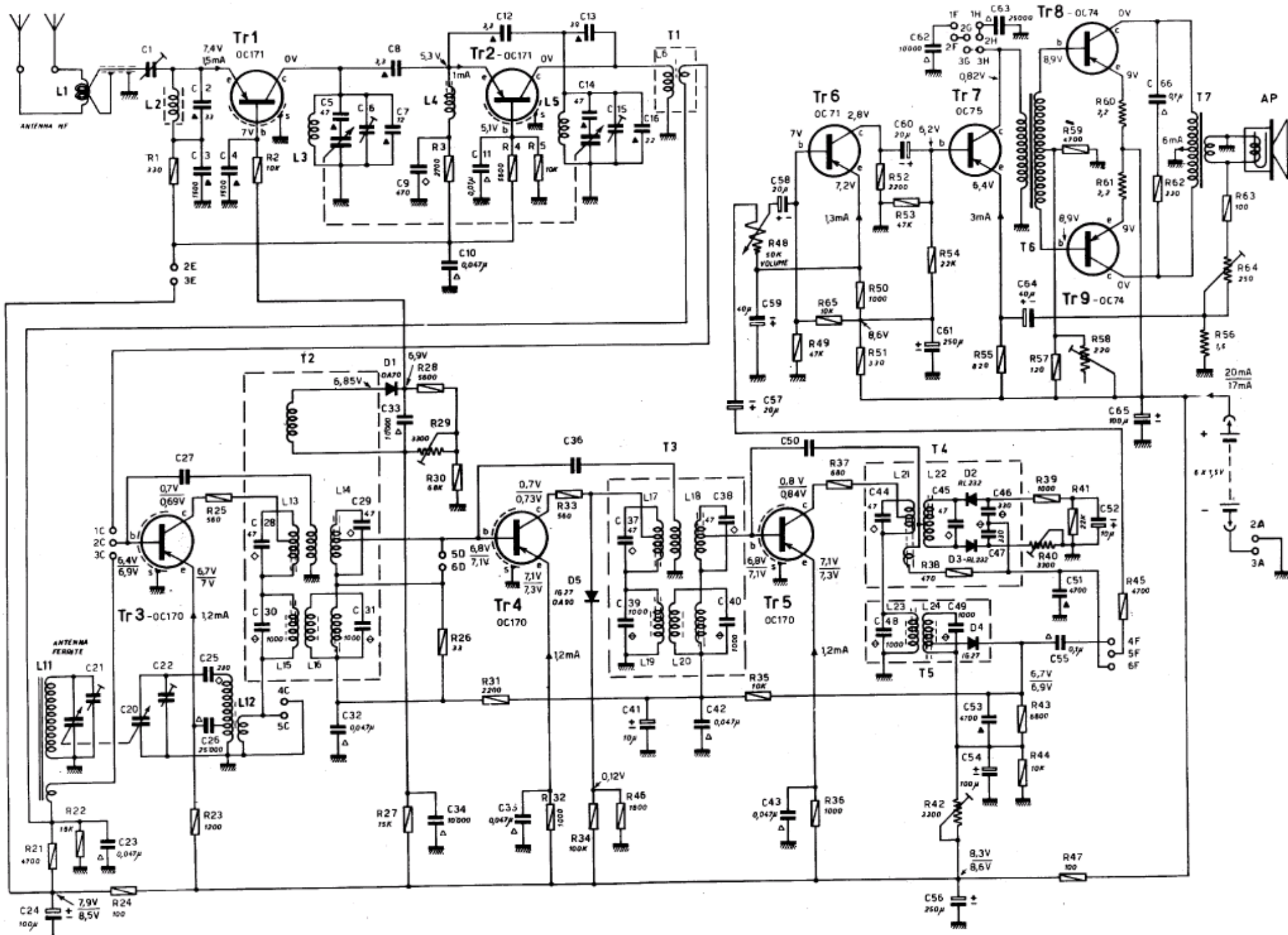
RADIORICEVITORE PHONOLA Mod. T 901
